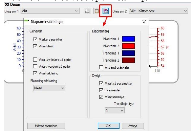
Bild 3. Rekommenderade diagraminställningar
