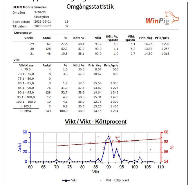
Bild 2. Rapporten Omgångsstatistik
