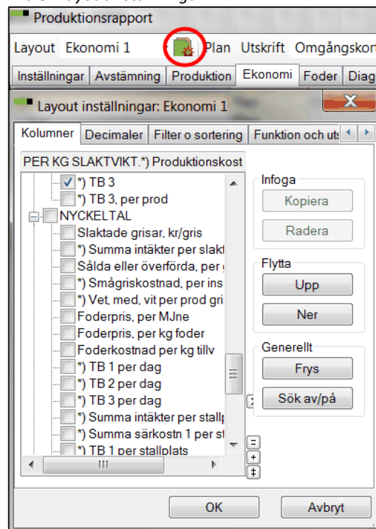
Bild 3. Layoutinställningar
