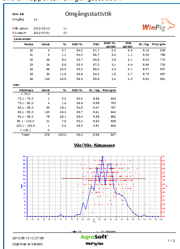
Bild 2. Rapporten Omgångsstatistik
