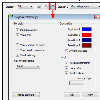
Bild 3. Rekommenderade diagraminställningar
