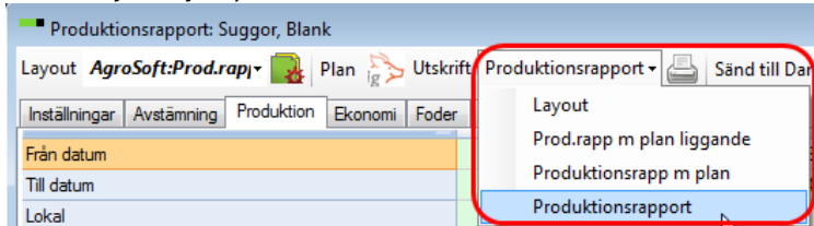
Bild 1. Välj utskriftslayout
