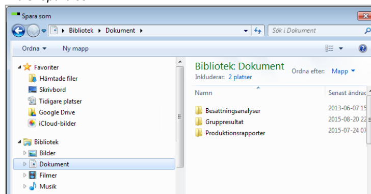
Bild 3. Spara som
