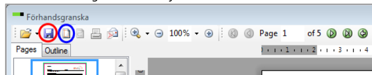
Bild 2. Förhandsgranska utskriften
